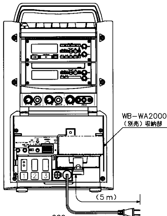
カバーを外した 背面図
