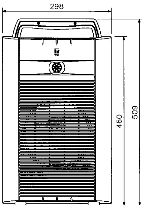
正面図
